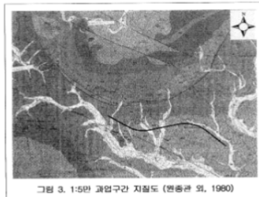
그림 3. 1:5만 과업구간 지질도 (원종관 외, 1980)
